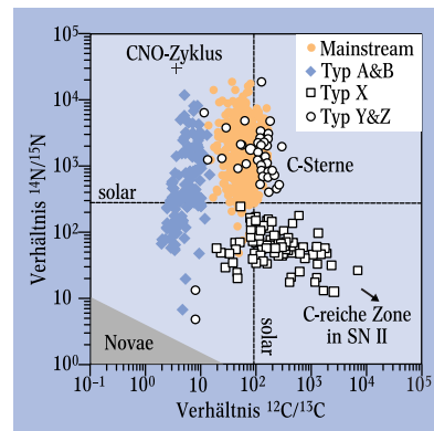
Abb. 5: Isotopensignaturen in präsolaren Staubkörnern: Die Kohlen- und Stickstoff-Isotopen- verhältnisse erlauben es, die erwarteten Ursprungs-Orte einzelner Körner zu charakterisie- ren. Die Typeinteil- lungen beruhen auf anderen Isoto- penverhältnissen.
