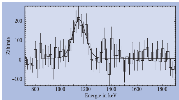
Abb. 2: Erstmals wurde radioaktives ^{44}\text{Ti} anhand seiner Gamma-Linie bei 1157 keV im Supernova-Überrest Cas A entdeckt. Das Spektrum wurde mit dem COMPTEL-Instrument auf dem Gamma-Observatorium COMPTON aufgenommen.
