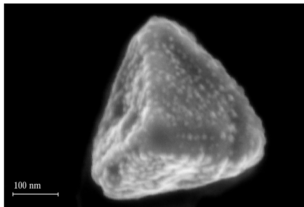
Abb. 4: Interstellares Staubkorn aus SiC
