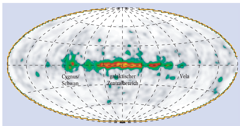
Abb. 3: Bild derzeitiger Nukleosynthese-Aktivität in der Milchstraßengalaxie. Die Karte zeigt den Himmel in 1,809 MeV-Emission von radioaktivem ^{26}\text{Al} (in galaktischen Koordinaten, die Intensität wächst von grün über rot nach gelb).
