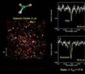
ESO/ISO (Photographie: Herberichs, van Dishoeck & Keesen)
