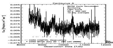
Fig. 1: BATSE Earth occultation data
